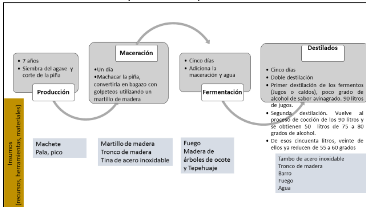
Esquema 1. Síntesis de producción de mezcal.
